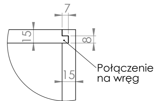
SZCZEGÓŁ C SKALA 2 : 5
